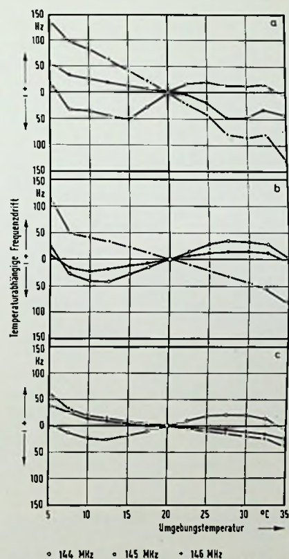
Der Temperaturgang der Frequenzen: Das Diagramm a wurde ohne die Diode D 3 aufgenommen. Mit D 3 wurden die als b bezeichneten Kurven erzielt. C-Diagramm zeigt die Bestwerte, nachdem C 1 ausgetauscht worden war.
