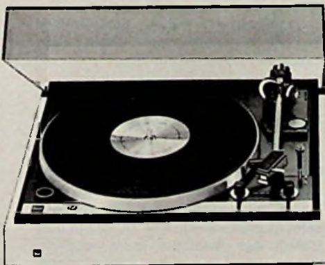
Manueller und automatischer HiFi-Plattenspieler Dual CS 701 W – Electronic Direct Drive.
