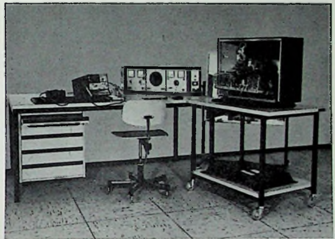
Die Abbildung zeigt einen Meß- und Prüfplatz mit hera-Arbeits- u. Labor-tisch LAT 2180, einen fahrbaren Unterschrank USS 2000 F, einen fahrbaren Spiegel und einen hera-Eckaufbau FR 75/1
